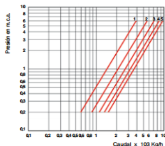
Pérdida de Carga Fluido: Agua a Temperatura 25°C
