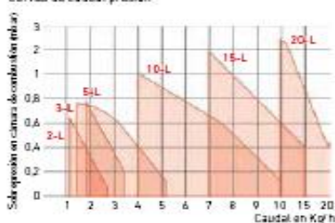
Curvas de caudal presión
